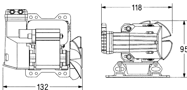
L: 132 mm B: 118 mm H: 95 mm C-C mått: 94x57 mm Håldia: 5 mm
